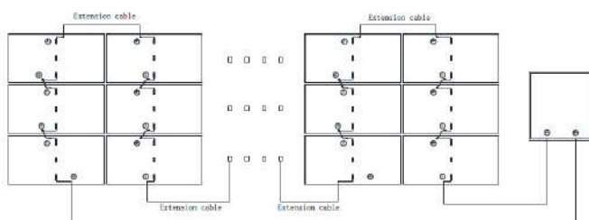
Rys. 9-3 Dzielona skrzynka łączeniowa przy module w położeniu środkowym dla kierunku poziomego
