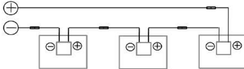
Rys. 10-1 Połączenie szeregowe
