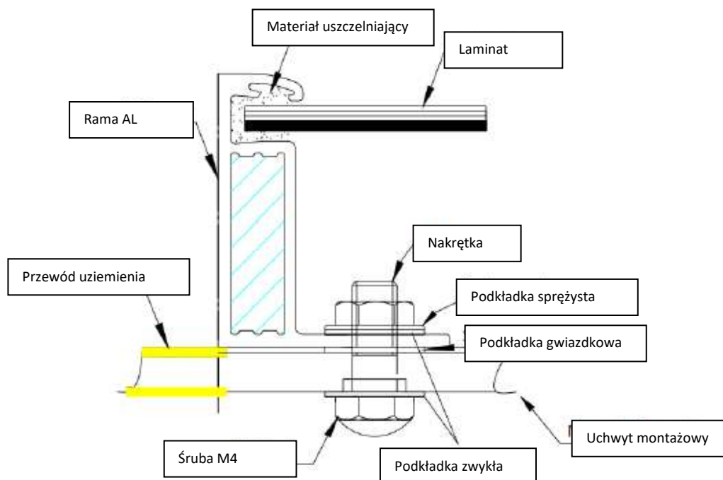
Rys. 11-1 Uziemienie
