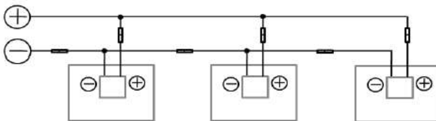
Rys. 10-2 Połączenie równoległe
